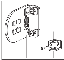
Натяжной трос
