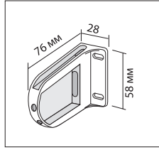
Кронштейн привода
